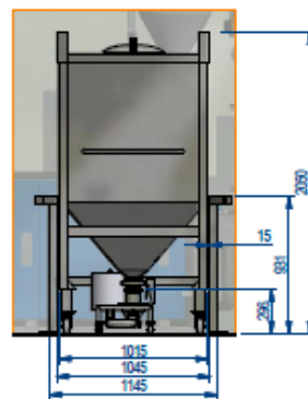
Detail B (1 : 35)
